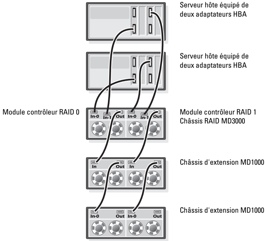
Figure 1-5. Câblage d'un cluster SAS à connexion directe
