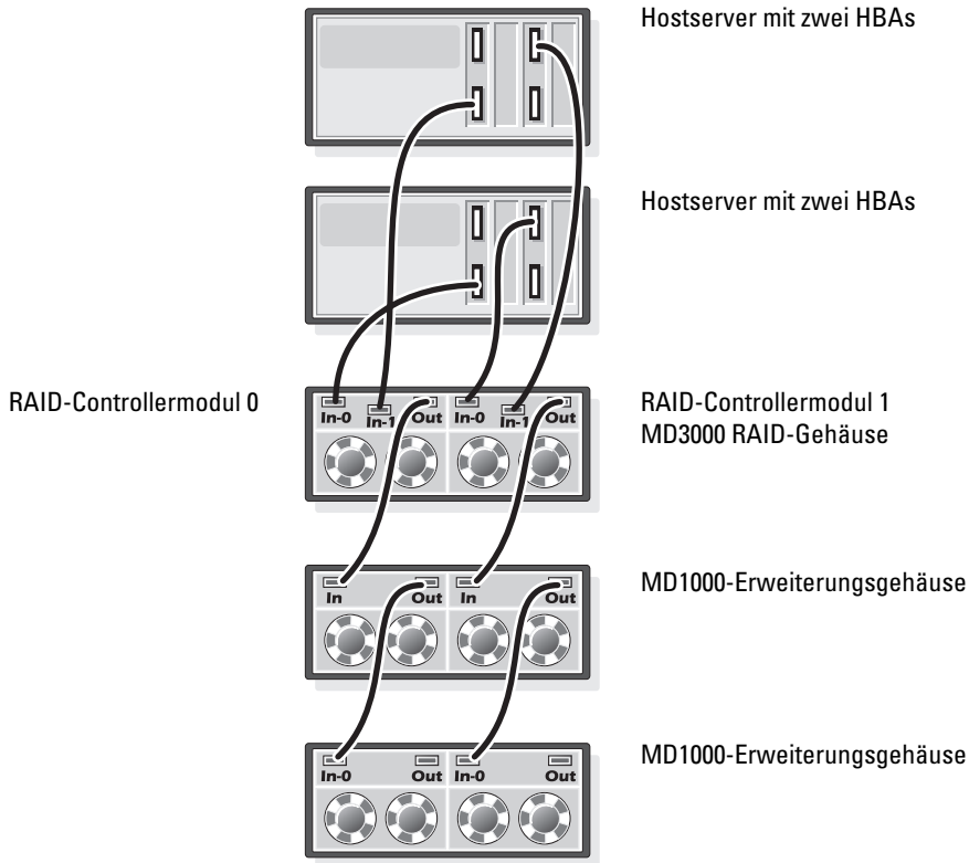
Abbildung 1-5. Direkt verbundenen SAS-Cluster verkabeln
