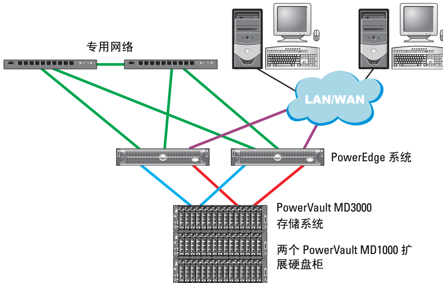
图 1-4. SAS 群集和 PowerVault MD3000 布线
