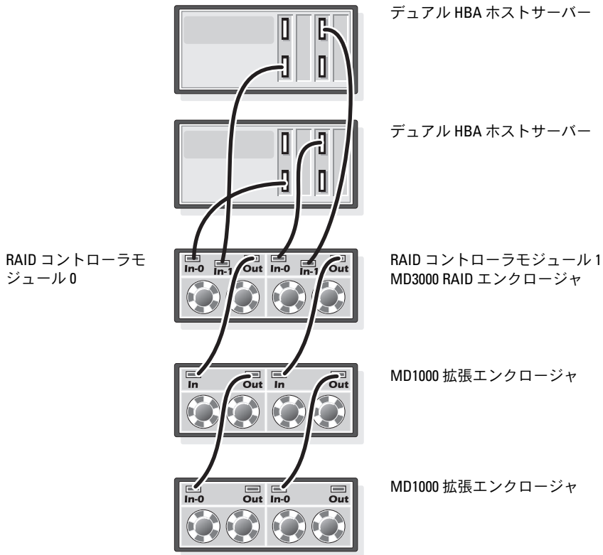
図 1-5 直接接続 SAS クラスタのケーブル接続
