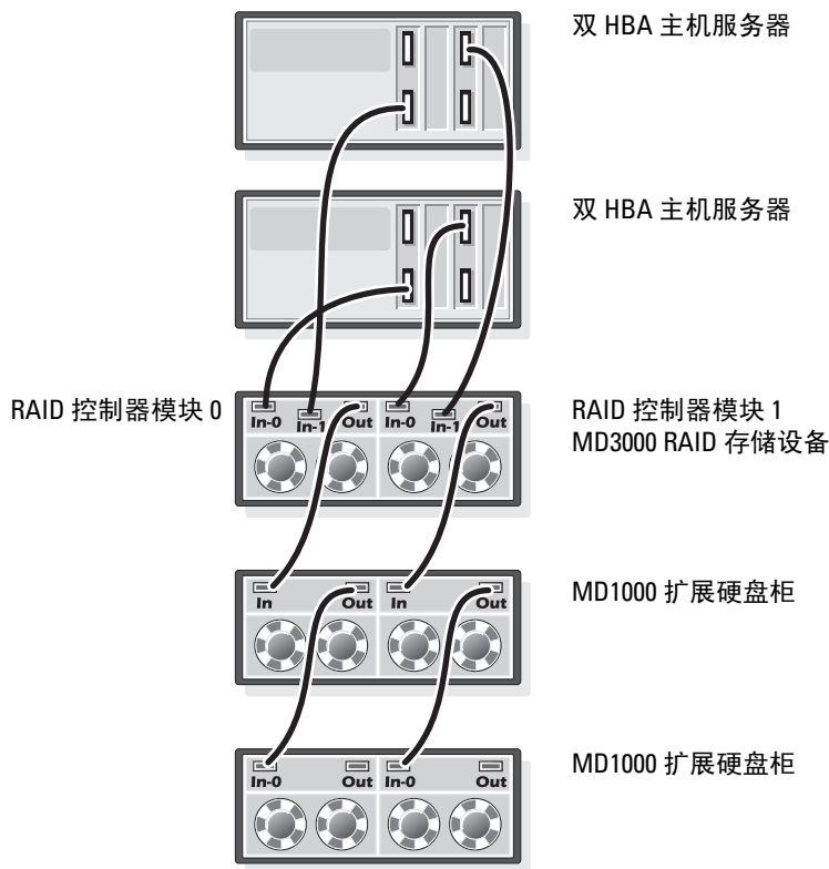
图 1-5. 直接连接 SAS 群集布线
