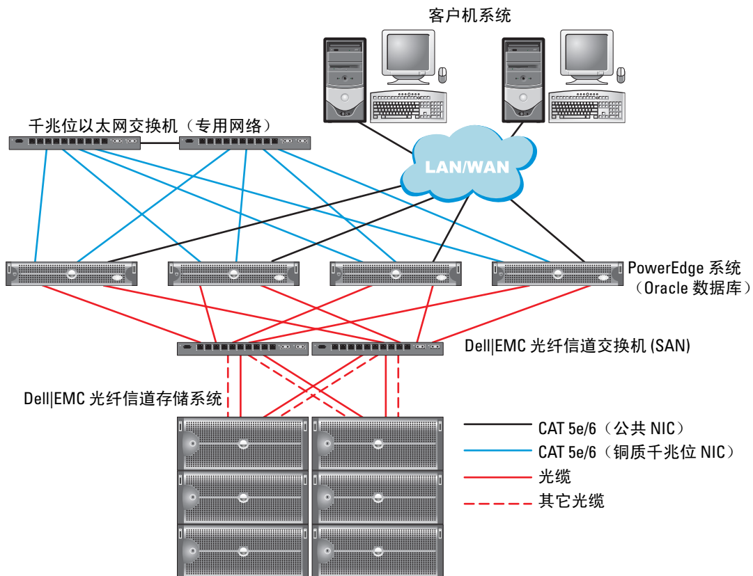
图 1-1. 光纤信道群集的硬件连接
