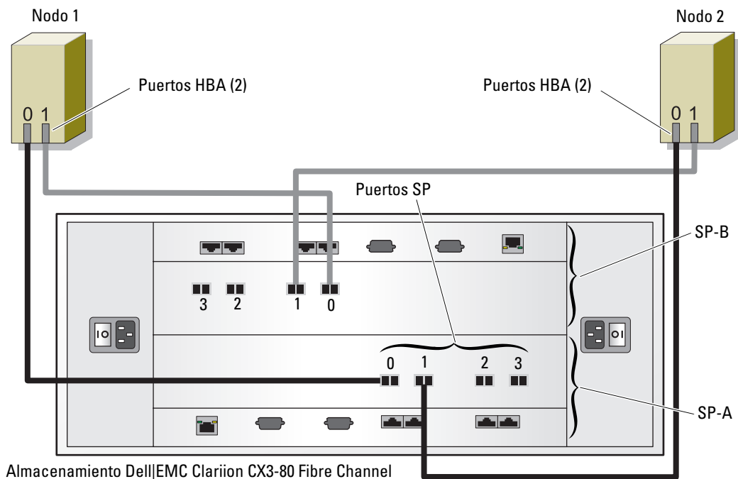
Ilustración 1-2. Cableado de un clúster Fibre Channel de conexión directa
