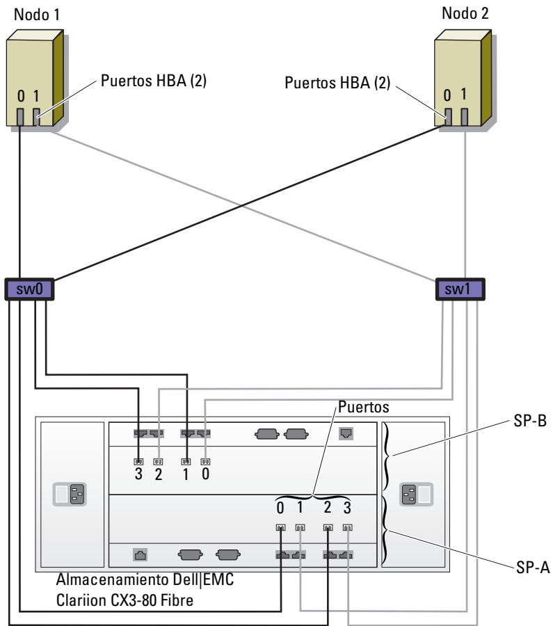
Ilustración 1-3. Cableado de un clúster Fibre Channel de conexión mediante SAN
