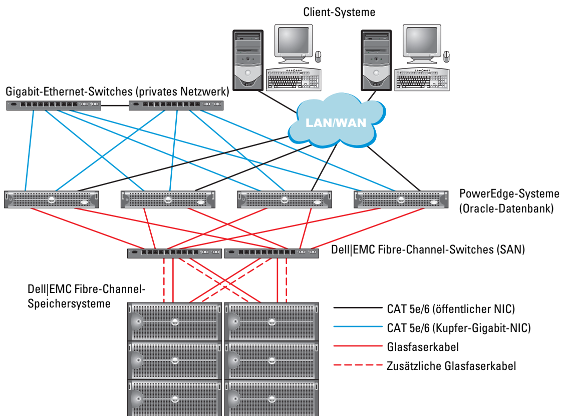
Abbildung 1-1. Hardwareverbindungen bei einem Fibre-Channel-Cluster
